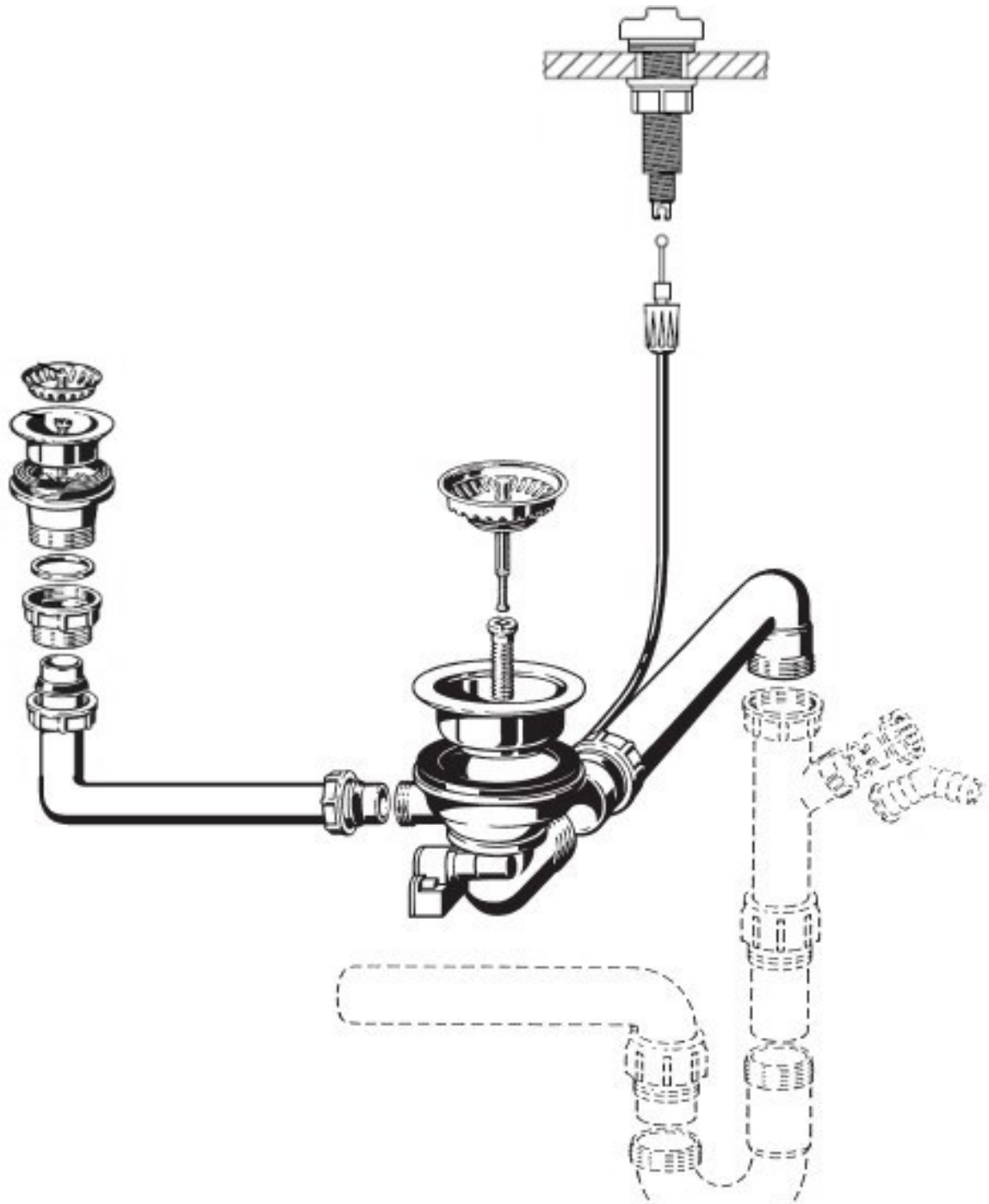
Ablaufgarnitur mit Excenterbetätigung 1 x 3 1/2"
